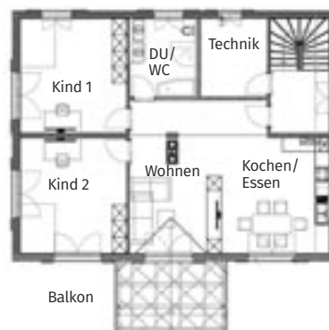
Obergeschoss
